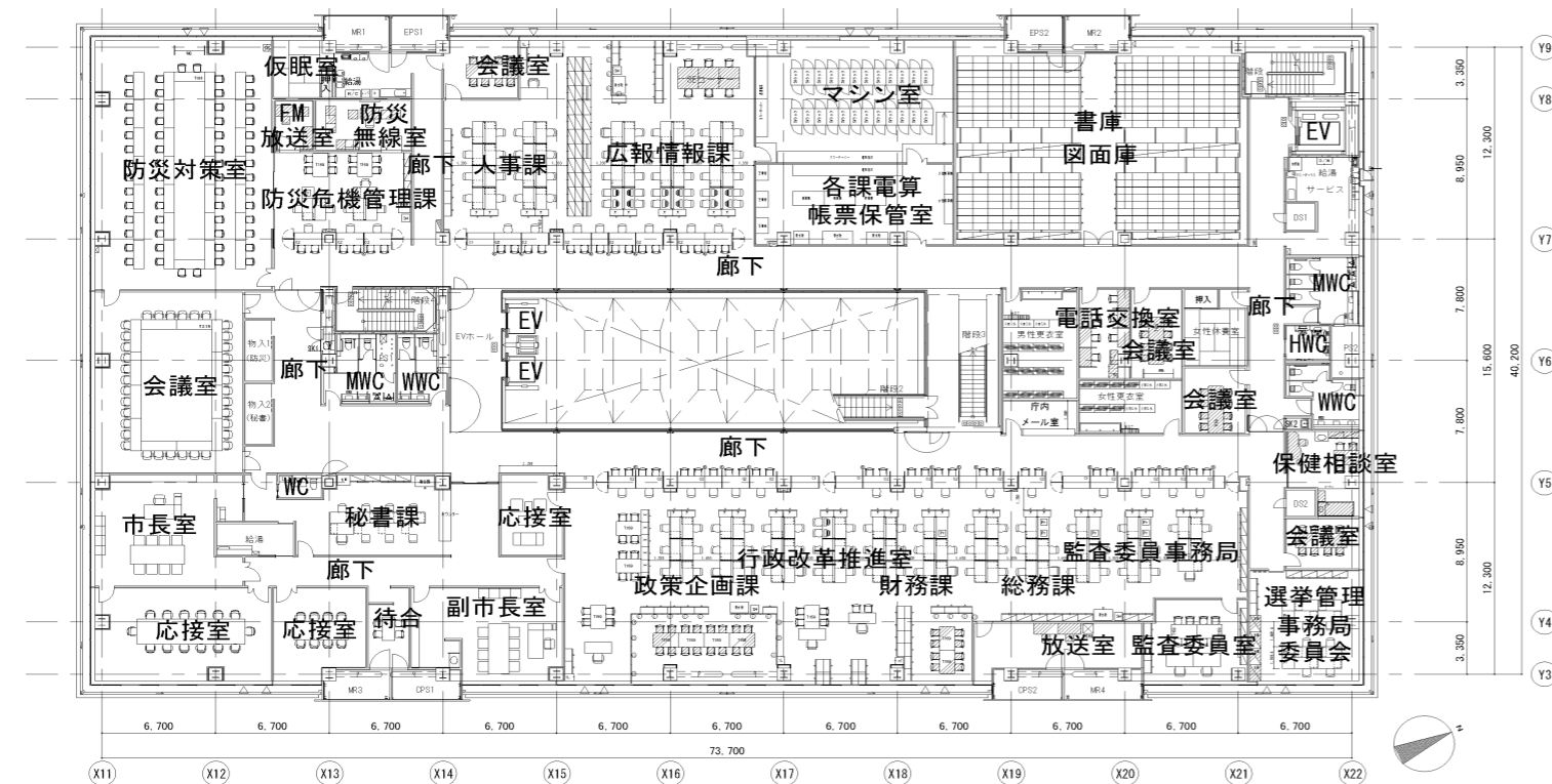
4階平面図
