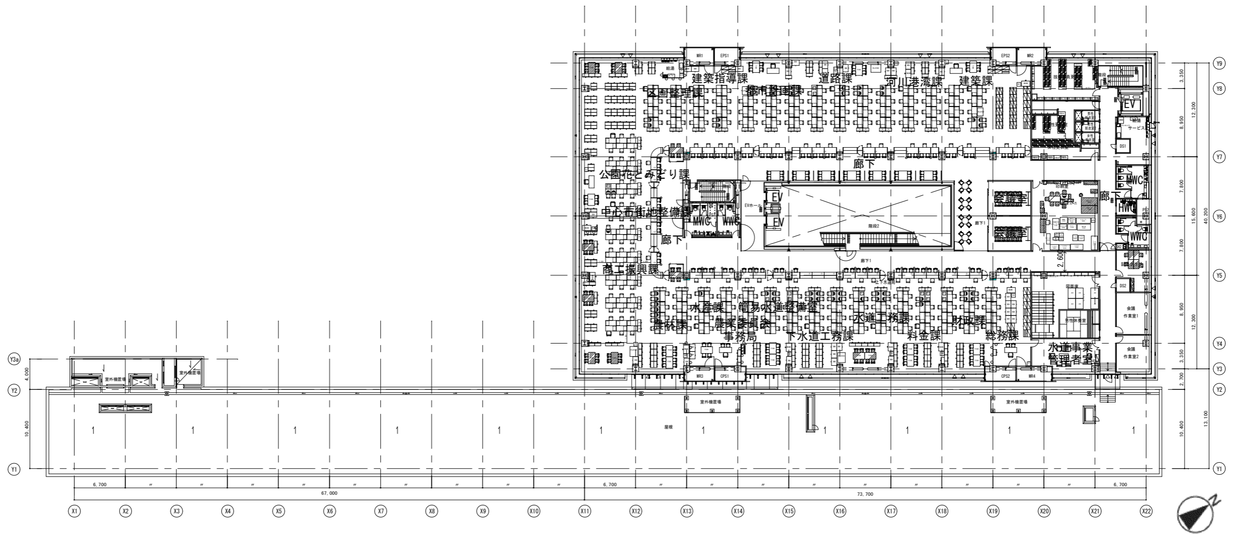
3階平面図
