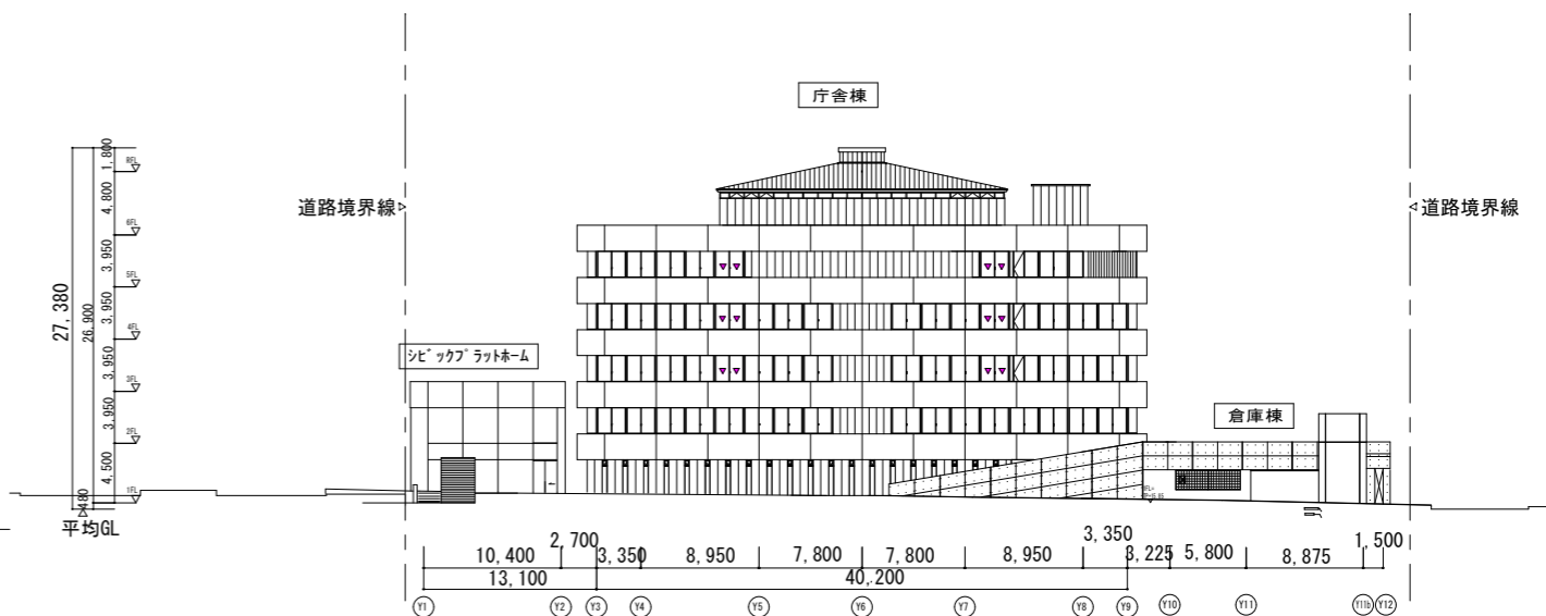
北側立面図
