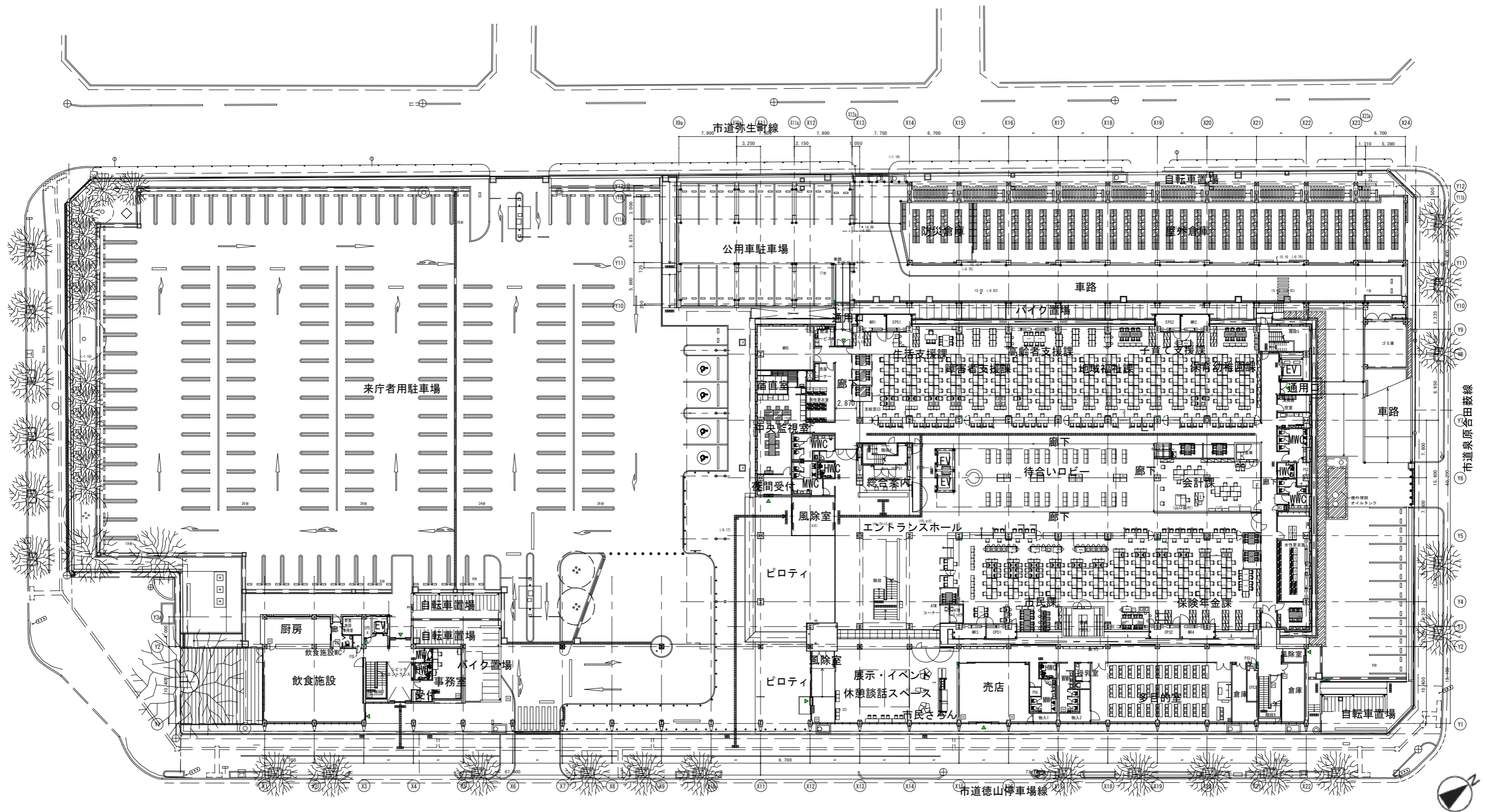
1階平面図
