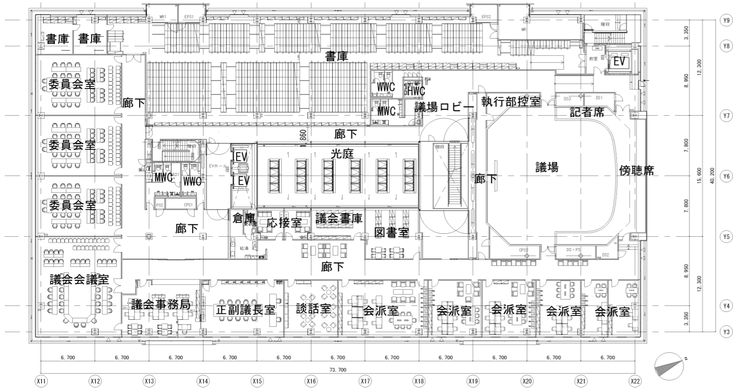
5階平面図
