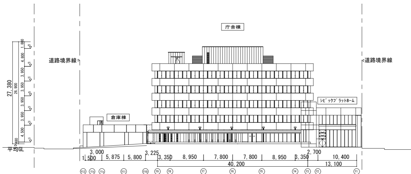
南側立面図
