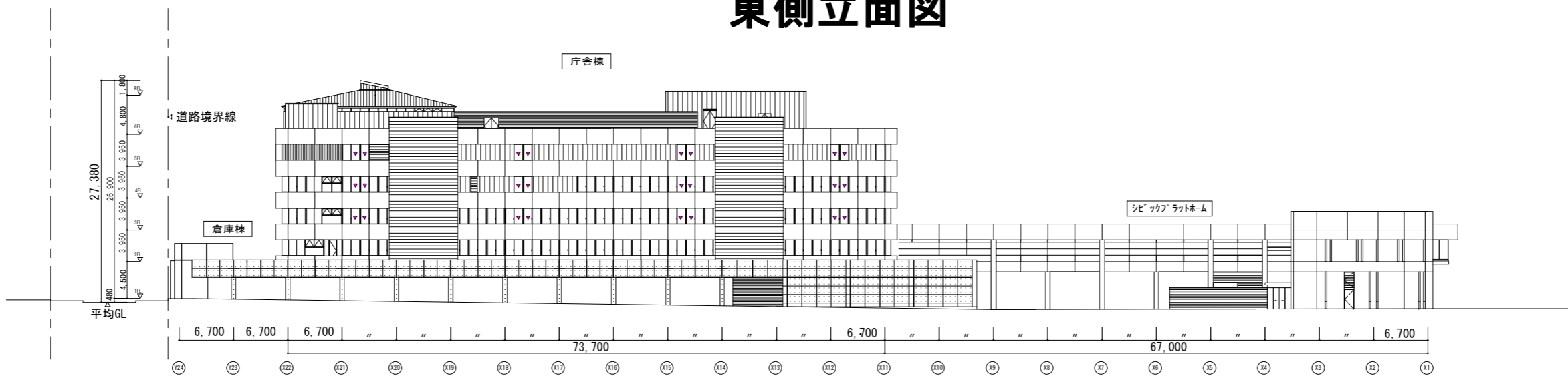
西側立面図
