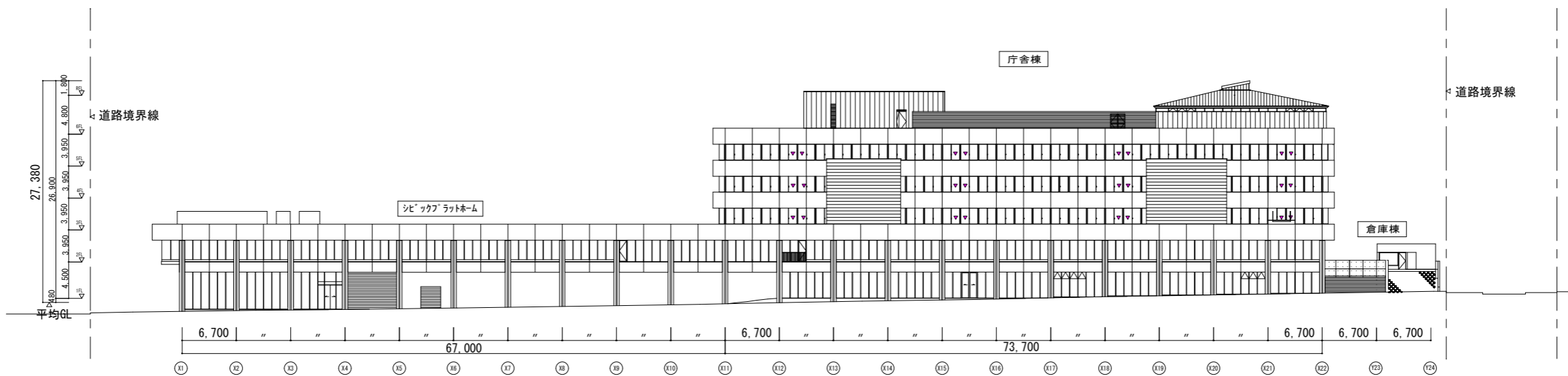
東側立面図
