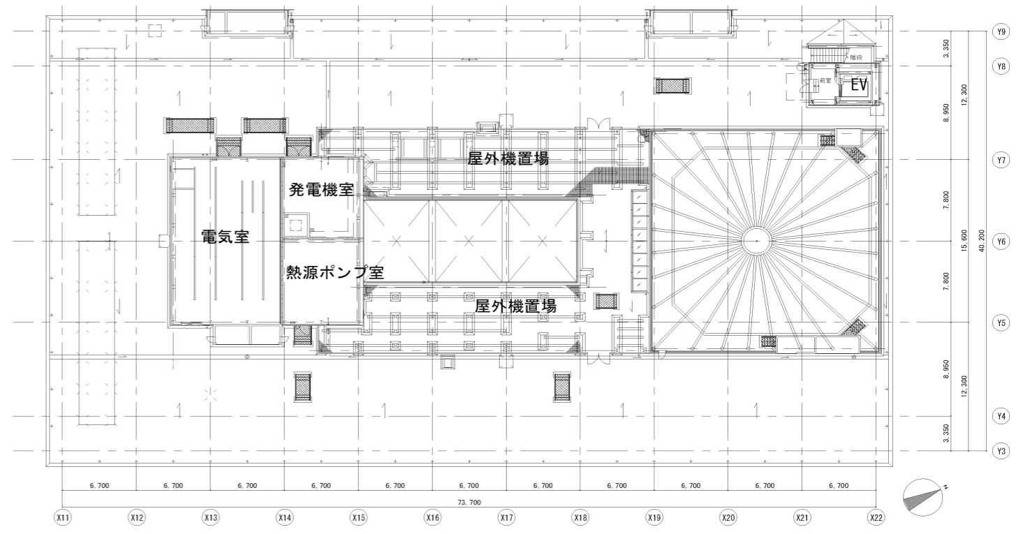
6階平面図
