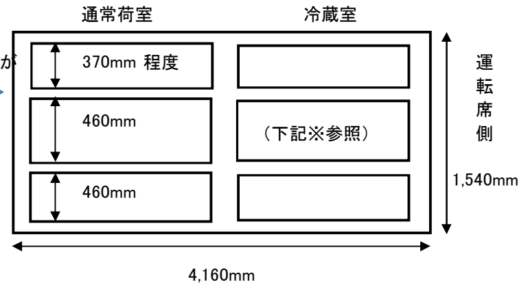
<荷台側面>
