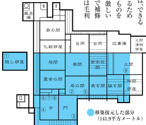
山田家本屋平面図
