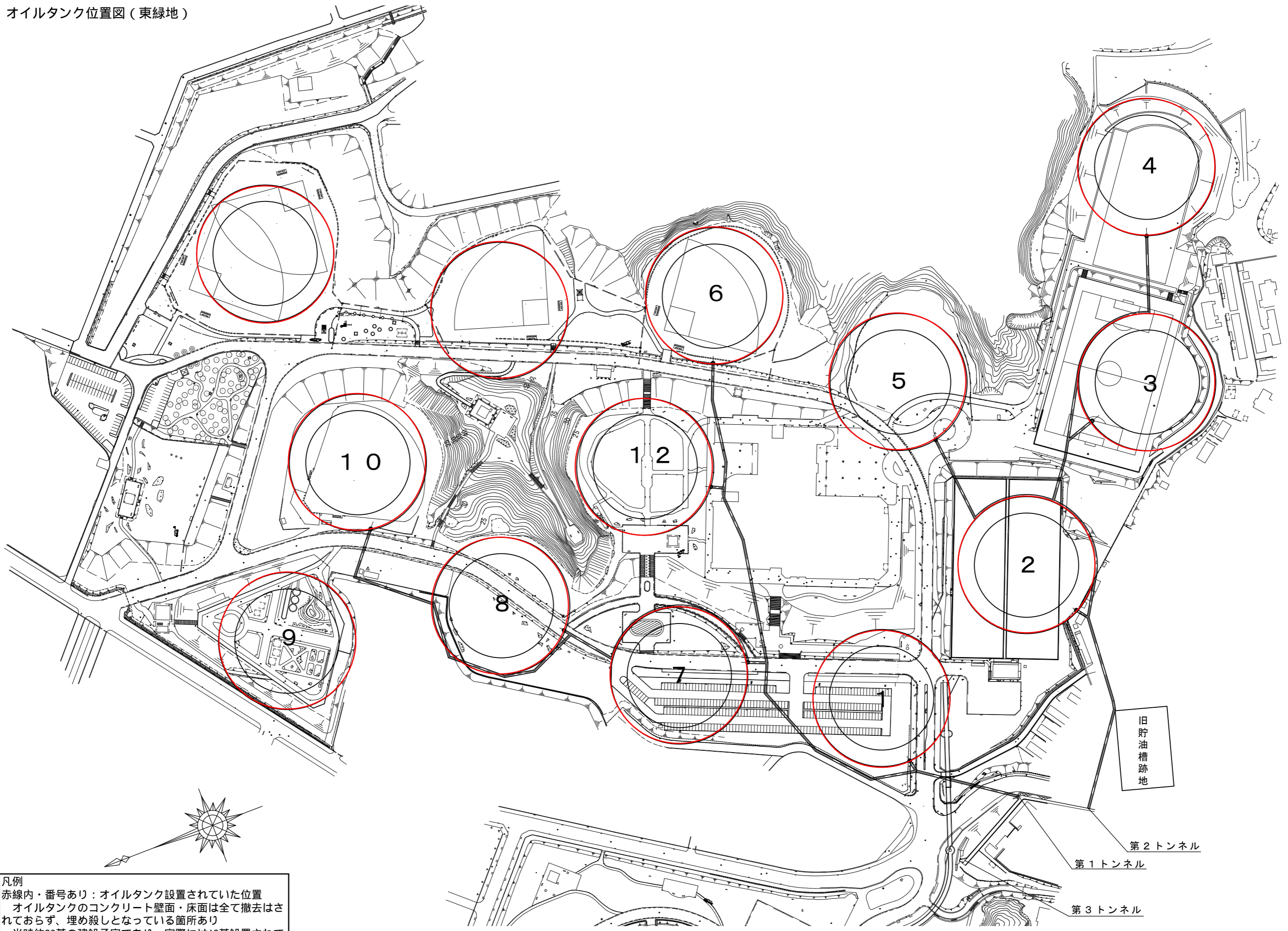
大迫田地下タンク (S=1:2500)
