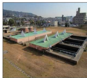
急速ろ過池
