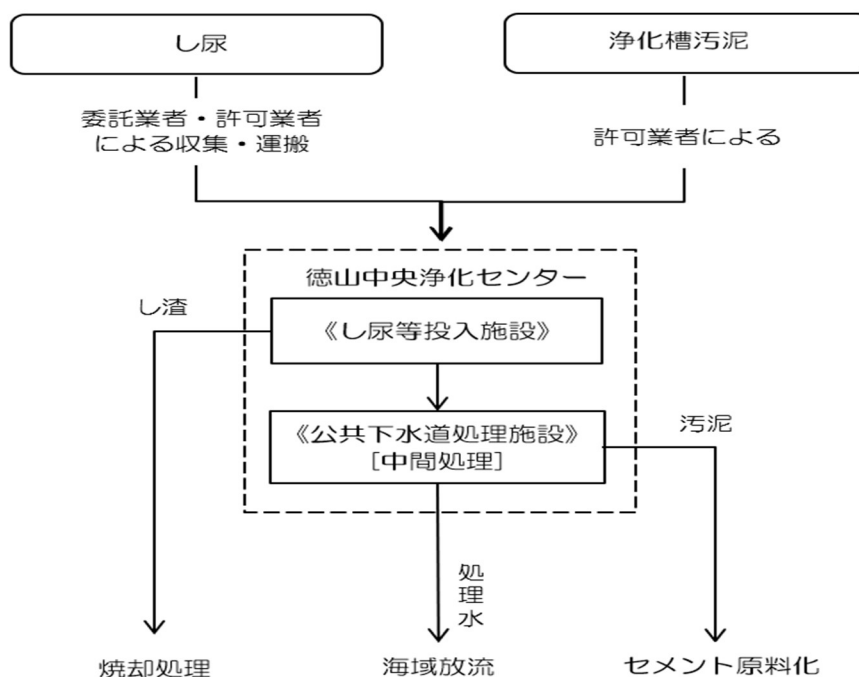
図表3-16 徳山中央浄化センターにおける処理工程(概略)
