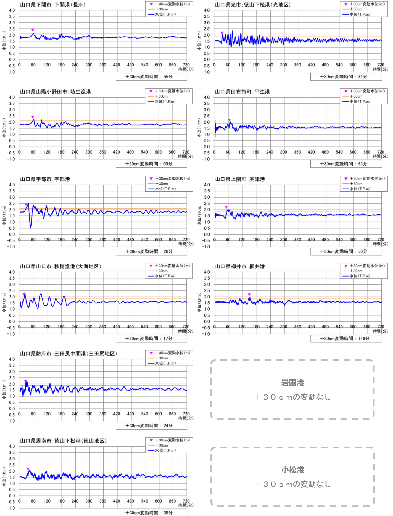
図一12(3) 海面変動+30m時間予測図(周防灘断層帯の地震)
