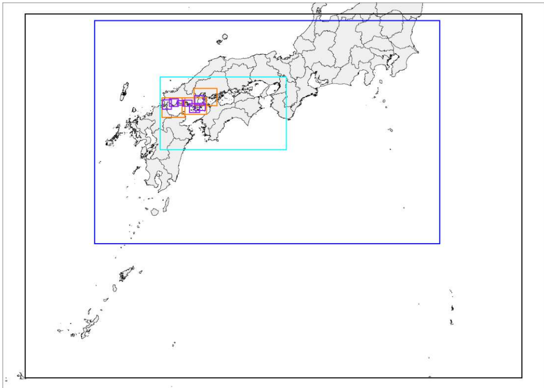
図-10 (1) 計算領域及び計算格子間隔 (2430m~30m)
