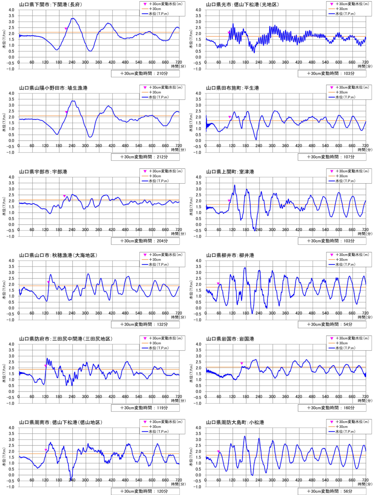
図一12 (1) 海面変動+30cm時間予測図 (南海トラフ巨大地震)
