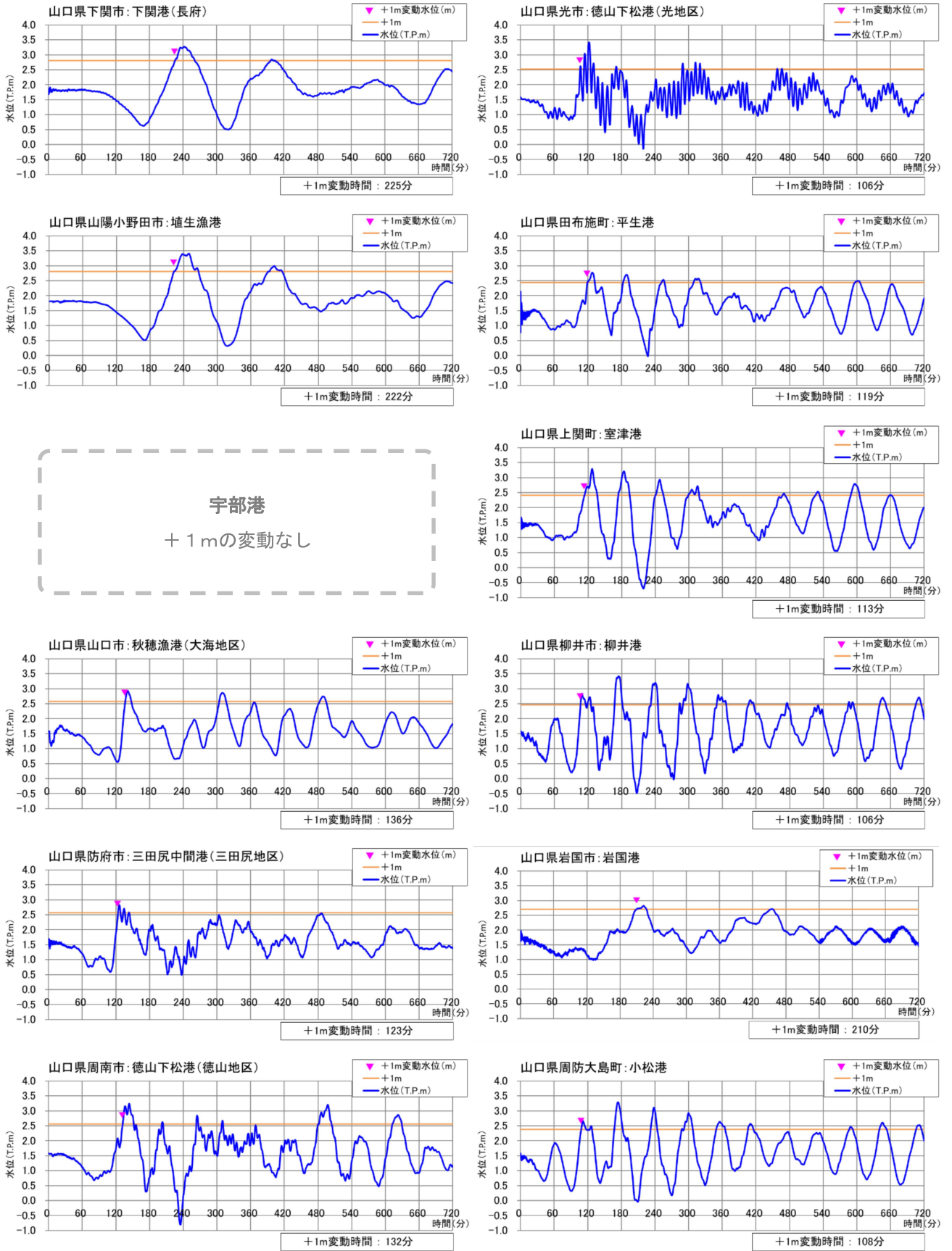
図一12(2) 海面変動+1m時間予測図(南海トラフ巨大地震)
