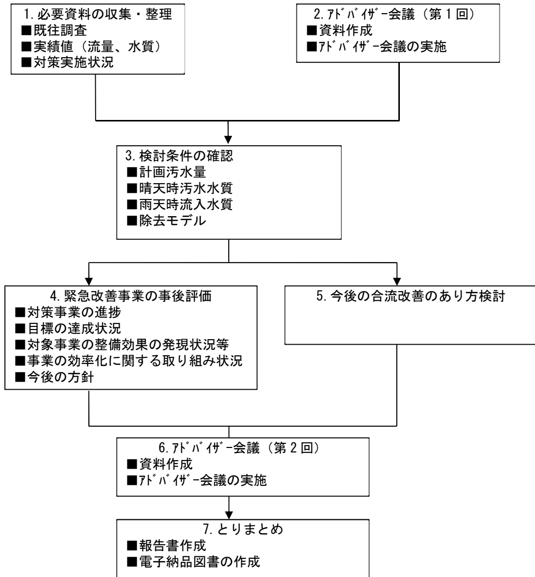
図 1-2 作業フロー
