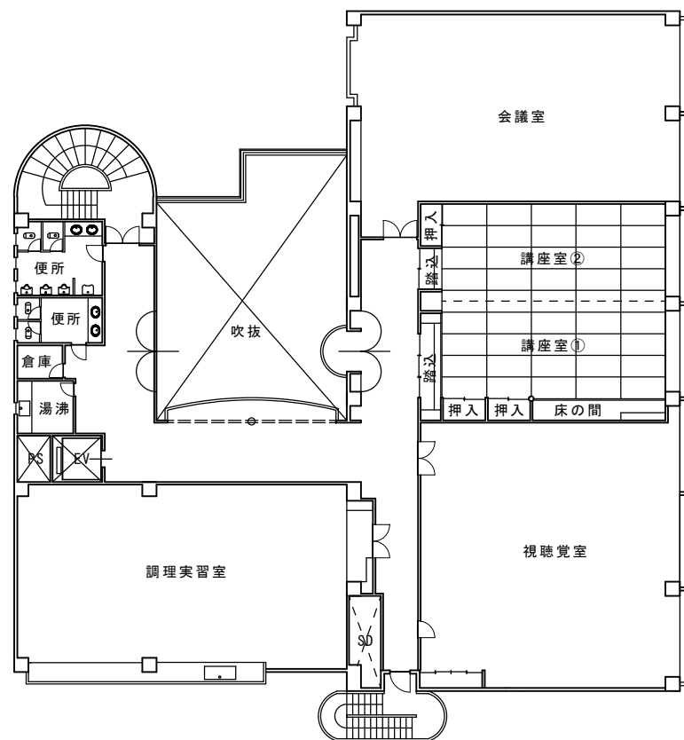
3階平面図
