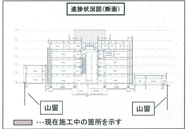
【横矢板設置完了(一部)】
