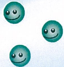
細菌類
