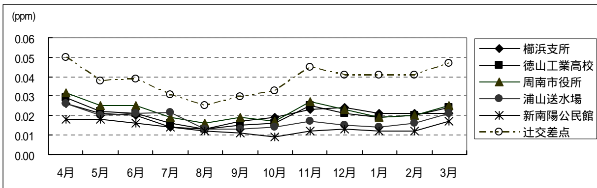
図 2 - 1 - 5 二酸化窒素の月別測定値 (月平均値)
