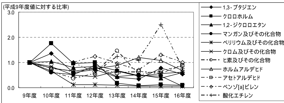
図2 - 1 - 18 環境基準および指針値のない有害大気汚染物質の推移（年平均値） ベンゾ[a]ピレン、酸化エチレンは平成11年度値に対する比率です。
