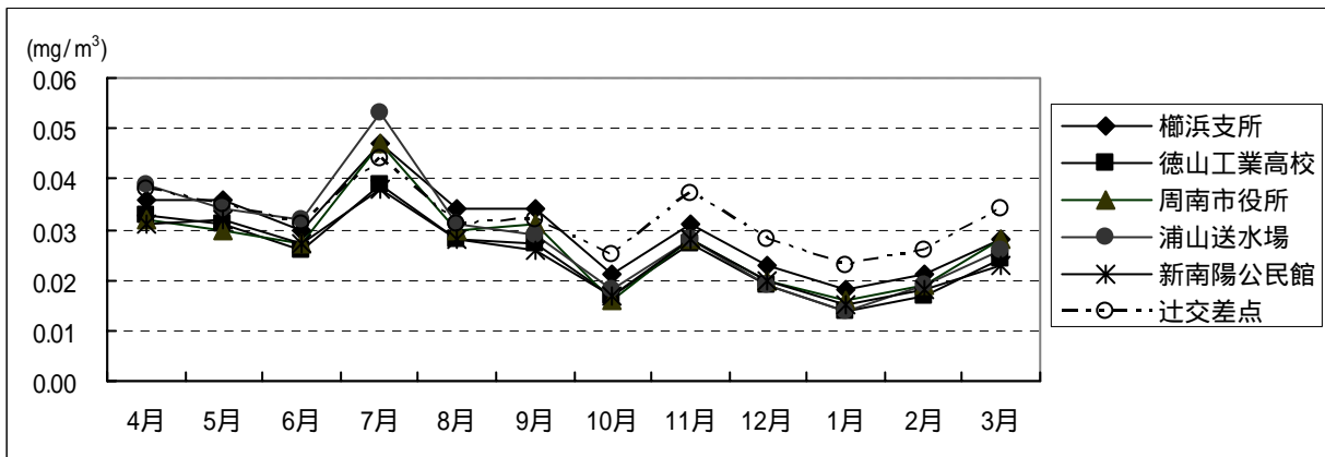
図2-1-9 浮遊粒子状物質の月別測定値(月平均値)
