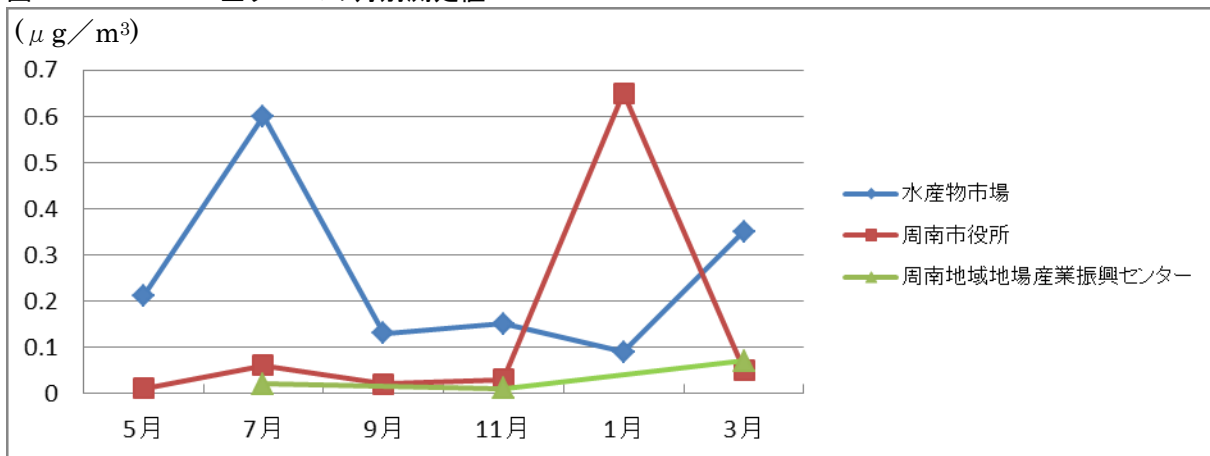
図2-1-32 全クロムの月別測定値
