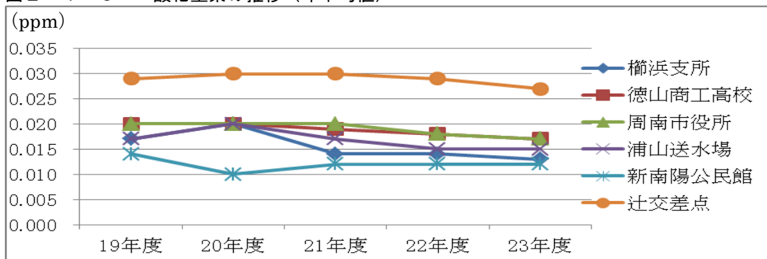
図2-1-6 二酸化窒素の推移(年平均値)
