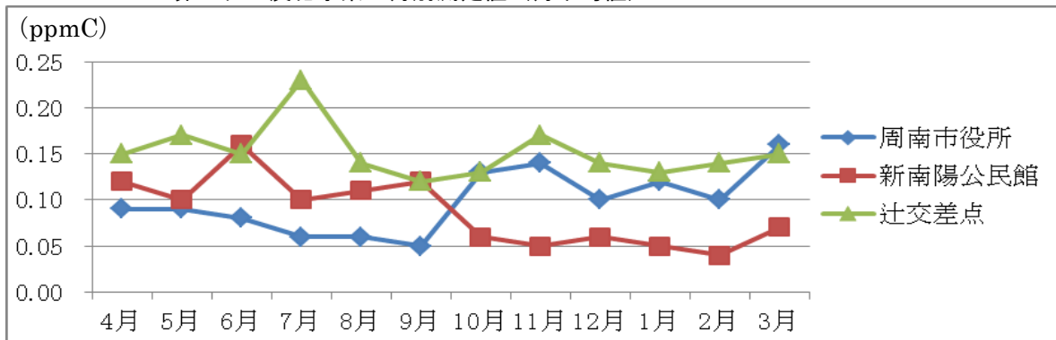
2-1-13 非メタン炭化水素の月別測定値 (月平均値)
