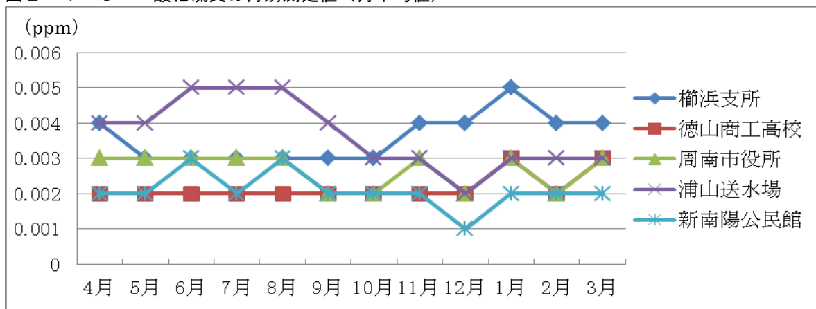
図 2-1-3 二酸化硫黄の月別測定値（月平均値）
