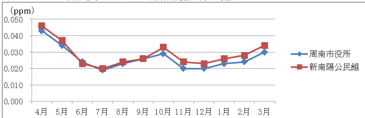
図2-1-11 光化学オキシダントの月別測定値（月平均値）
