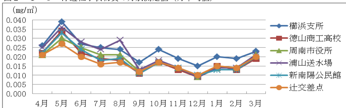
図2-1-9 浮遊粒子状物質の月別測定値（月平均値）
