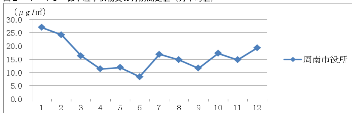
図2-1-15 微小粒子状物質の月別測定値(月平均値)
