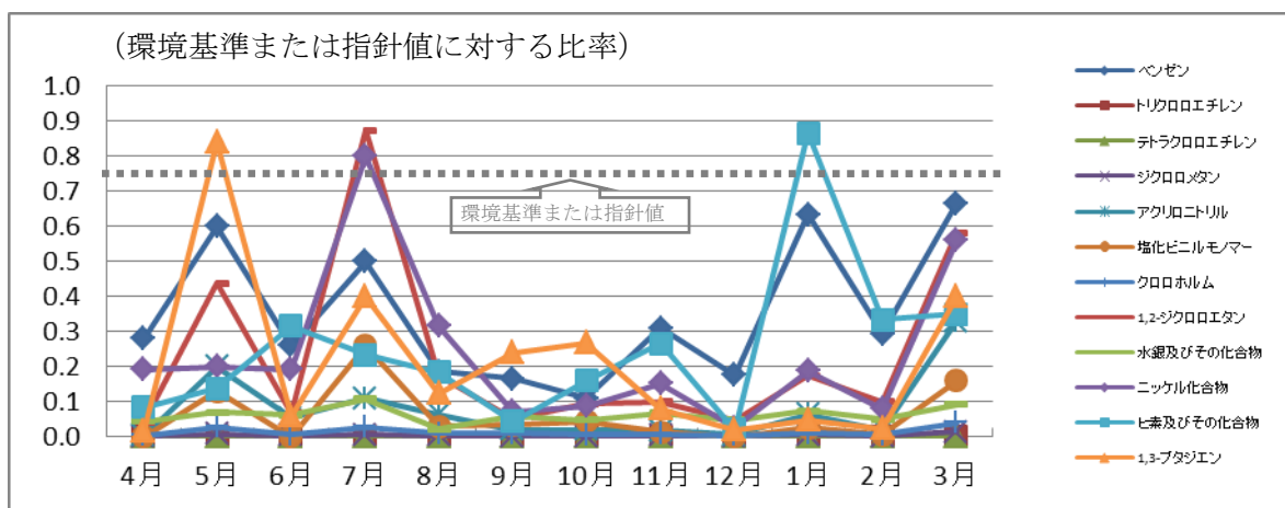
図 2-1-16 環境基準または指針値のある有害大気汚染物質の月別測定値
