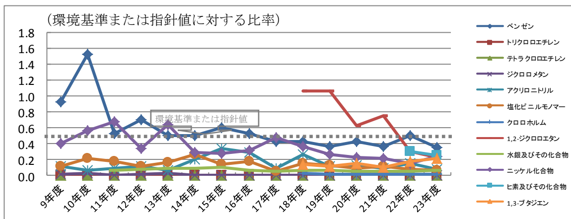
図 2-1-17 環境基準または指針値のある有害大気汚染物質の推移（年平均値）
