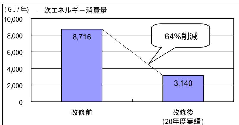
図3-5-2 市営路外駐車場のESCO事業の効果
