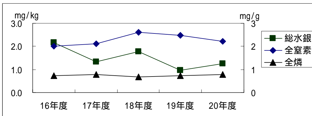
図2-2-9 経年変化の状況 (単位：総水銀はmg/kg、全窒素、全燐はmg/g)
