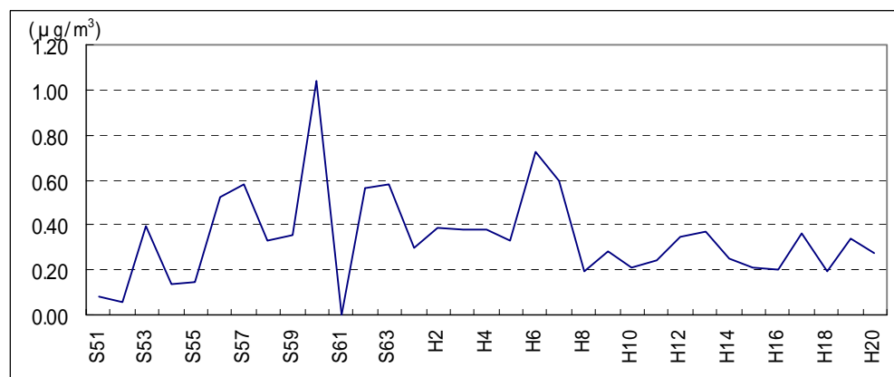
図 2 - 1 - 3 8 大気中のマグネシウム濃度の推移
