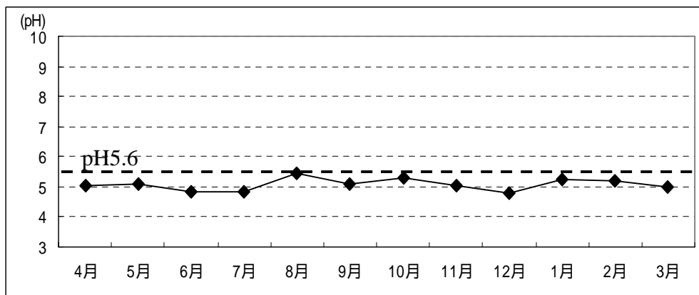
図 2 - 1 - 2 8 雨水の pH 月別測定値 (月平均値 1) )
