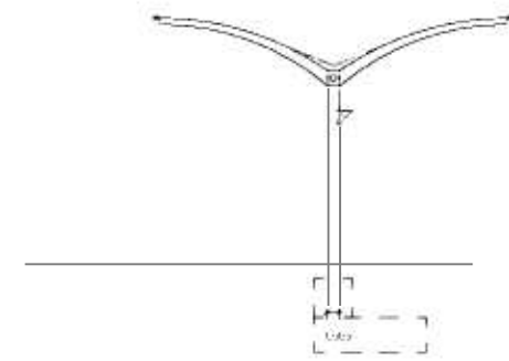
B-B'断面図
