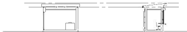
A-A' 断面图
