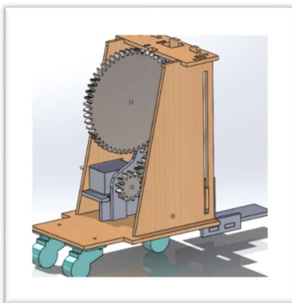
ロボットを 後ろ側から見た様子
