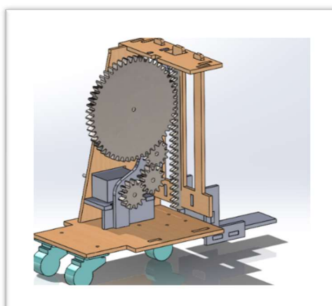
中が見えるように壁を外した様子 歯車と縦のギザギザの組み合わせが ラック・ピニオン機構
