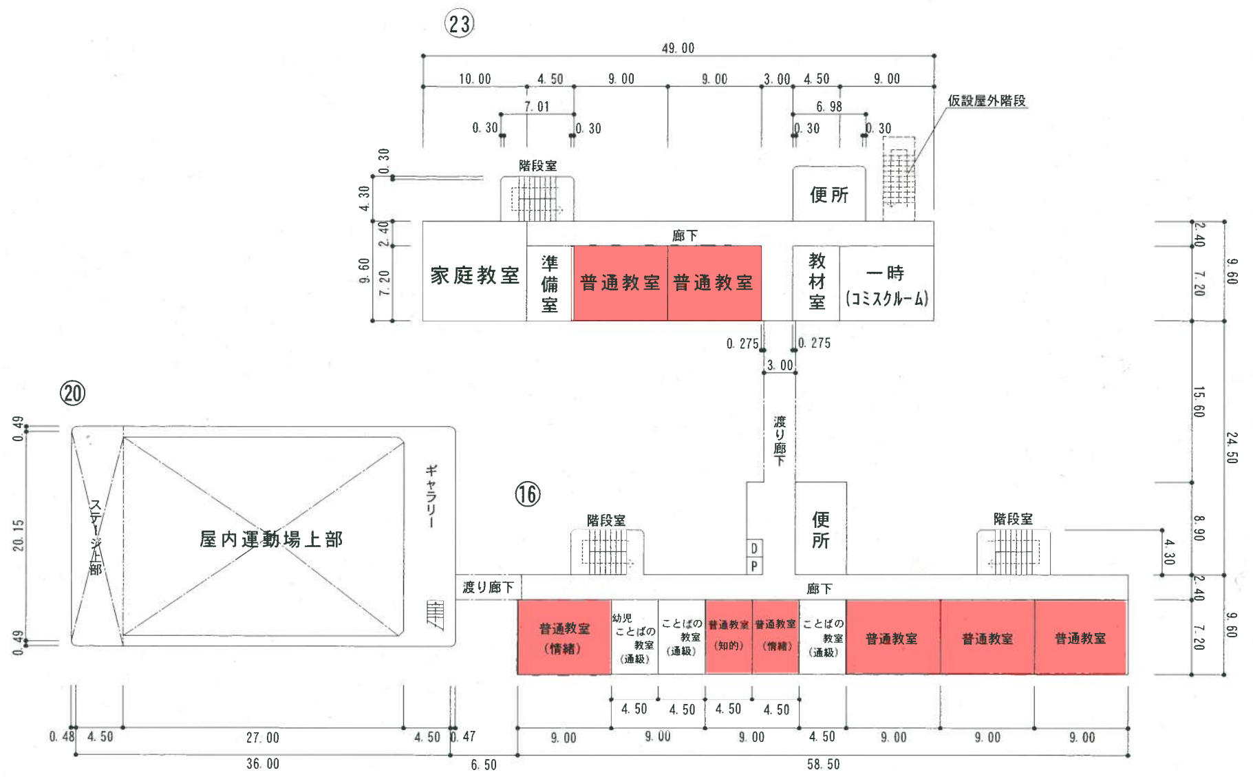
2階平面図
